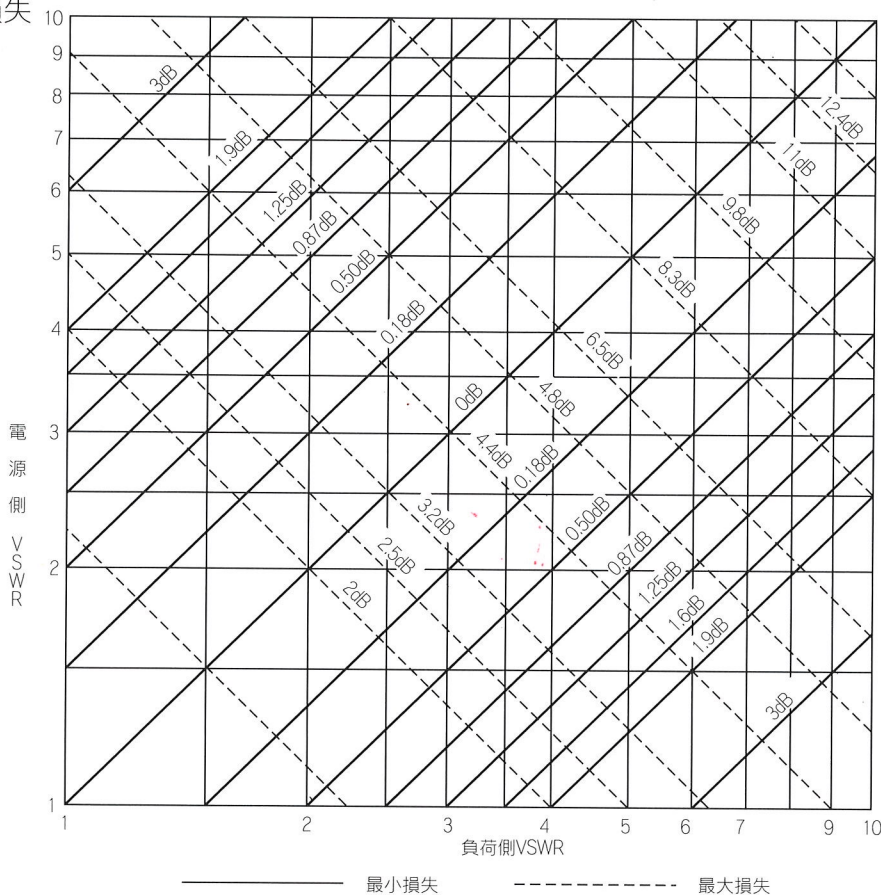
二つの不整合によって合成されるVSWRの最大値・最小値
