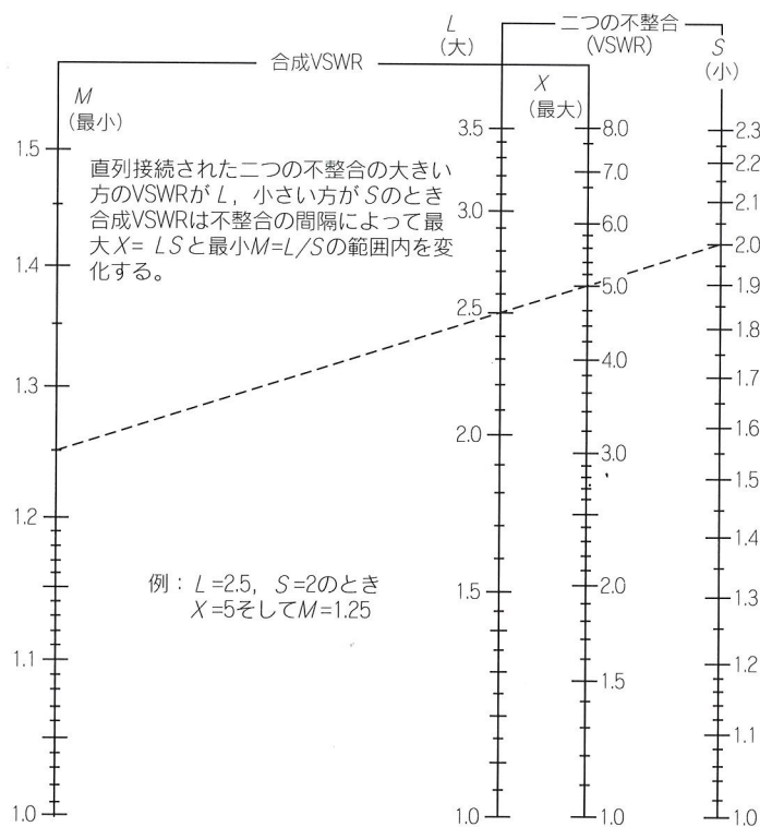
二つの不整合によって合成されるVSWRの最大値・最小値
